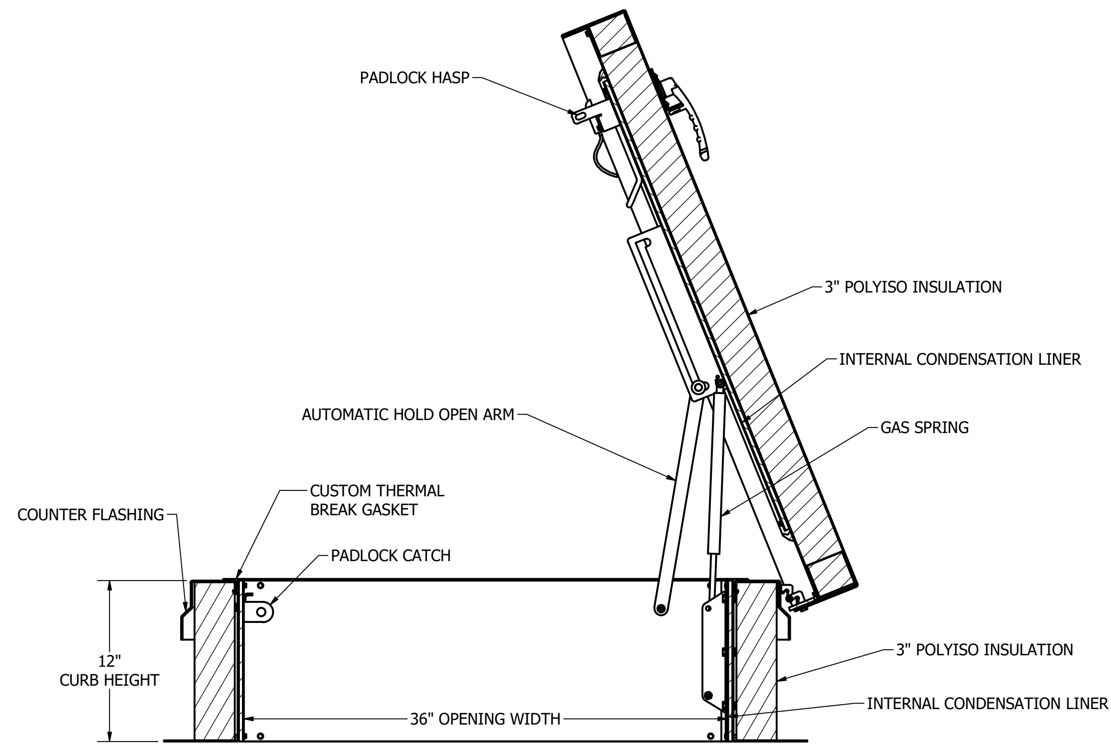
SECTION A-A SCALE 0.14 : 1
